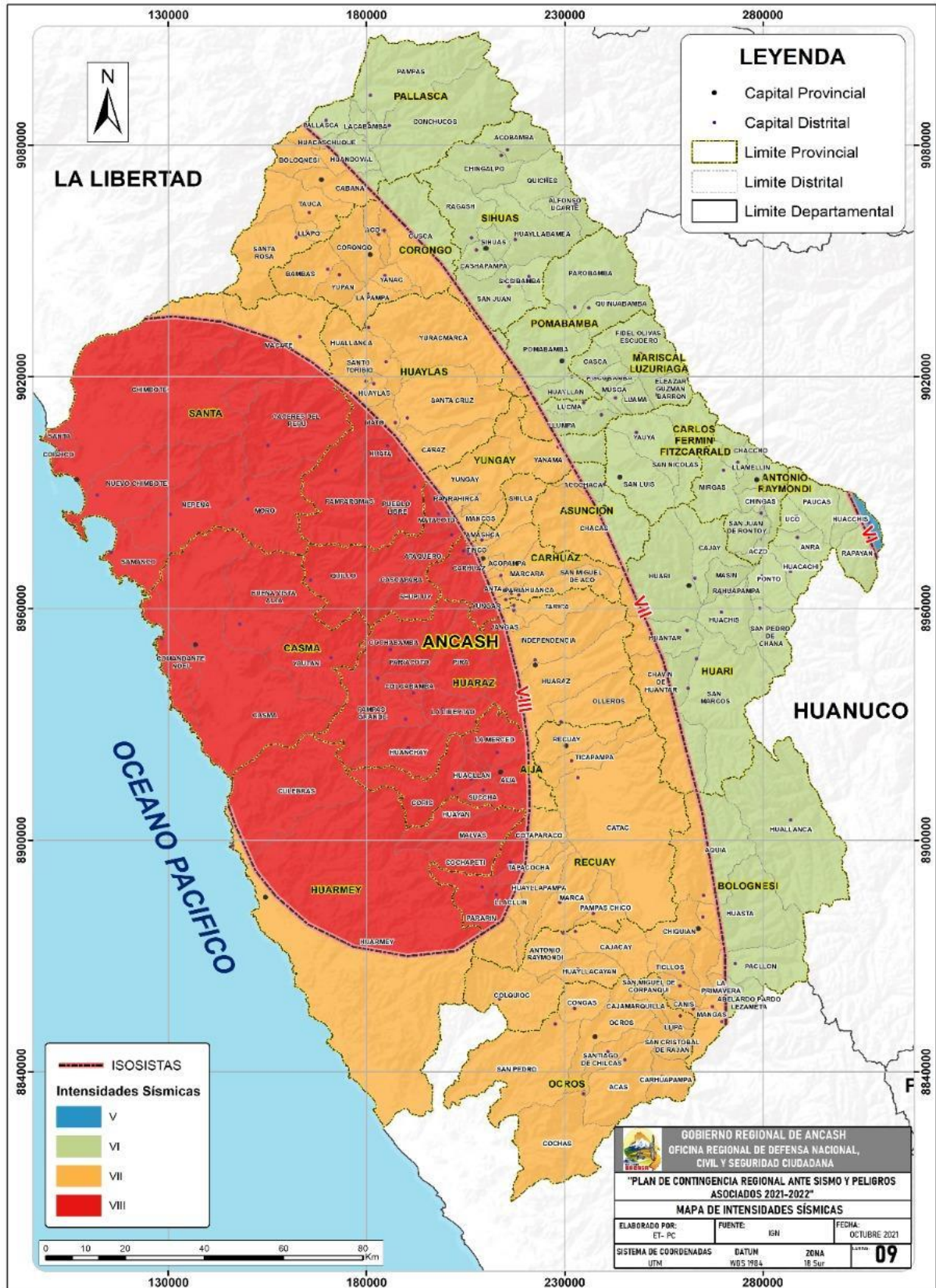
Mapa 35. Ancash: Intensidades Sísmicas
