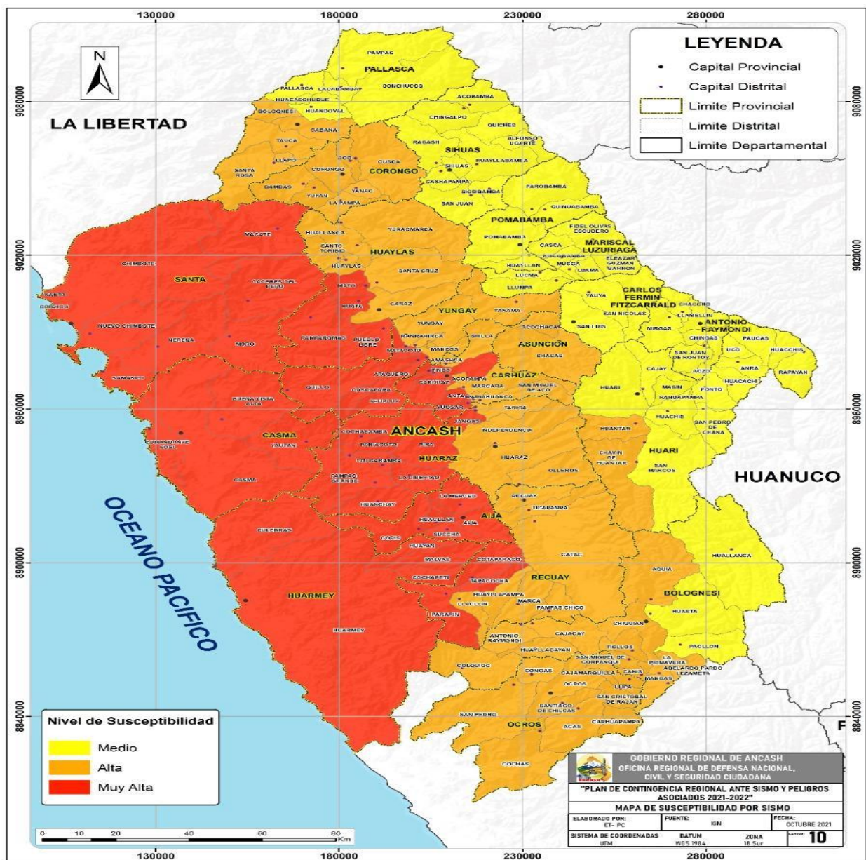
Mapa 36. Ancash: Susceptibilidad ante sismos en el Departamento de Ancash
