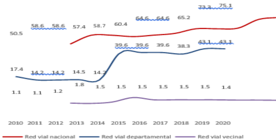
Gráfica 184. Ancash: Avance de Asfaltado de carreteras en la región
