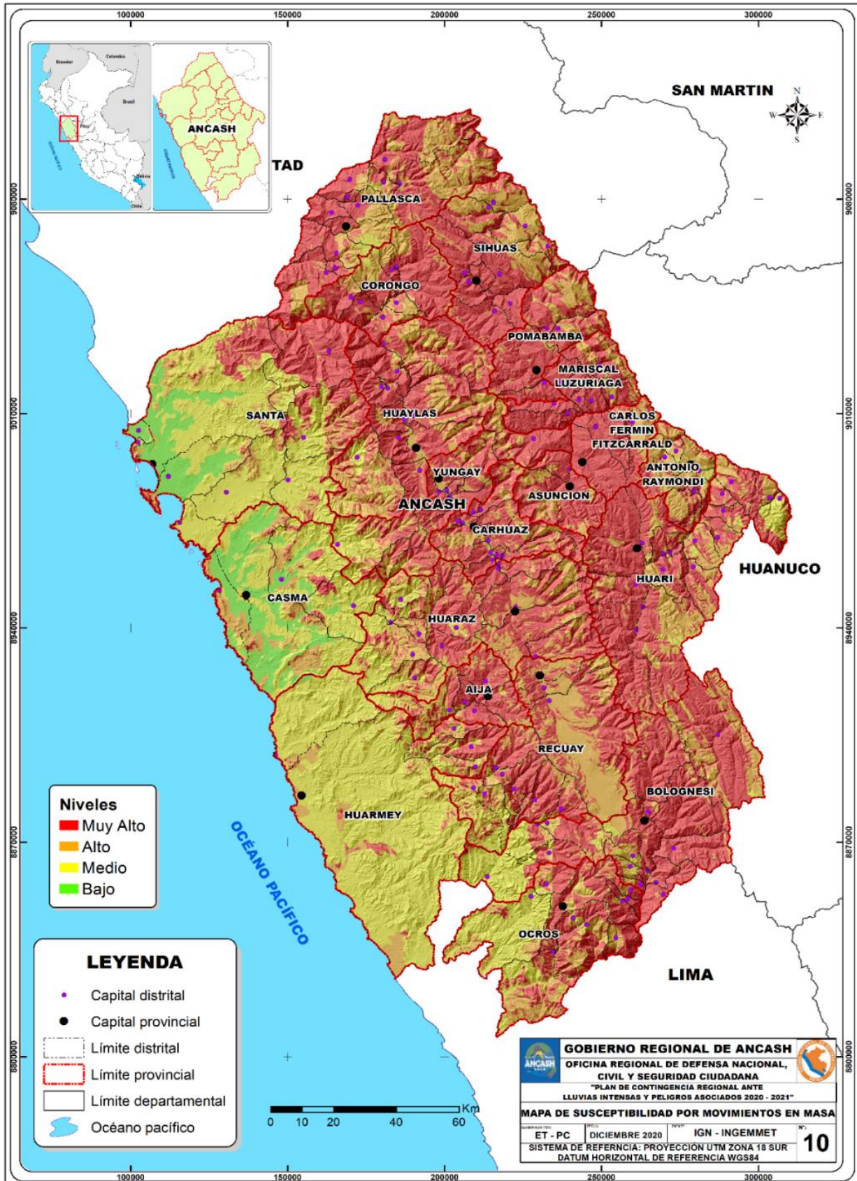
Mapa 38. Ancash: Susceptibilidad por movimientos en masa
