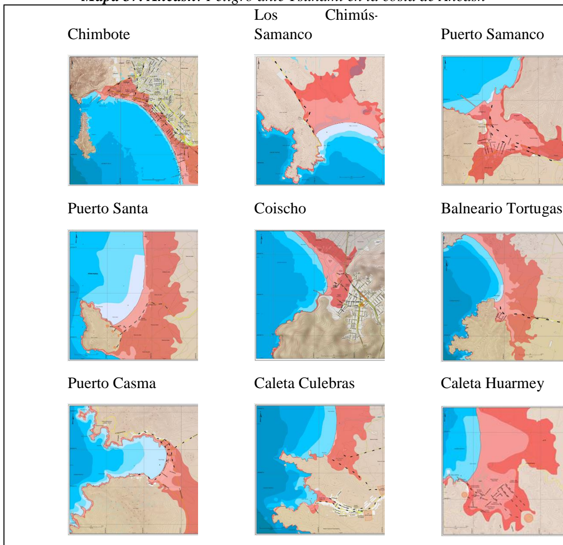
Mapa 37. Ancash: Peligro ante Tsunami en la costa de Ancash
