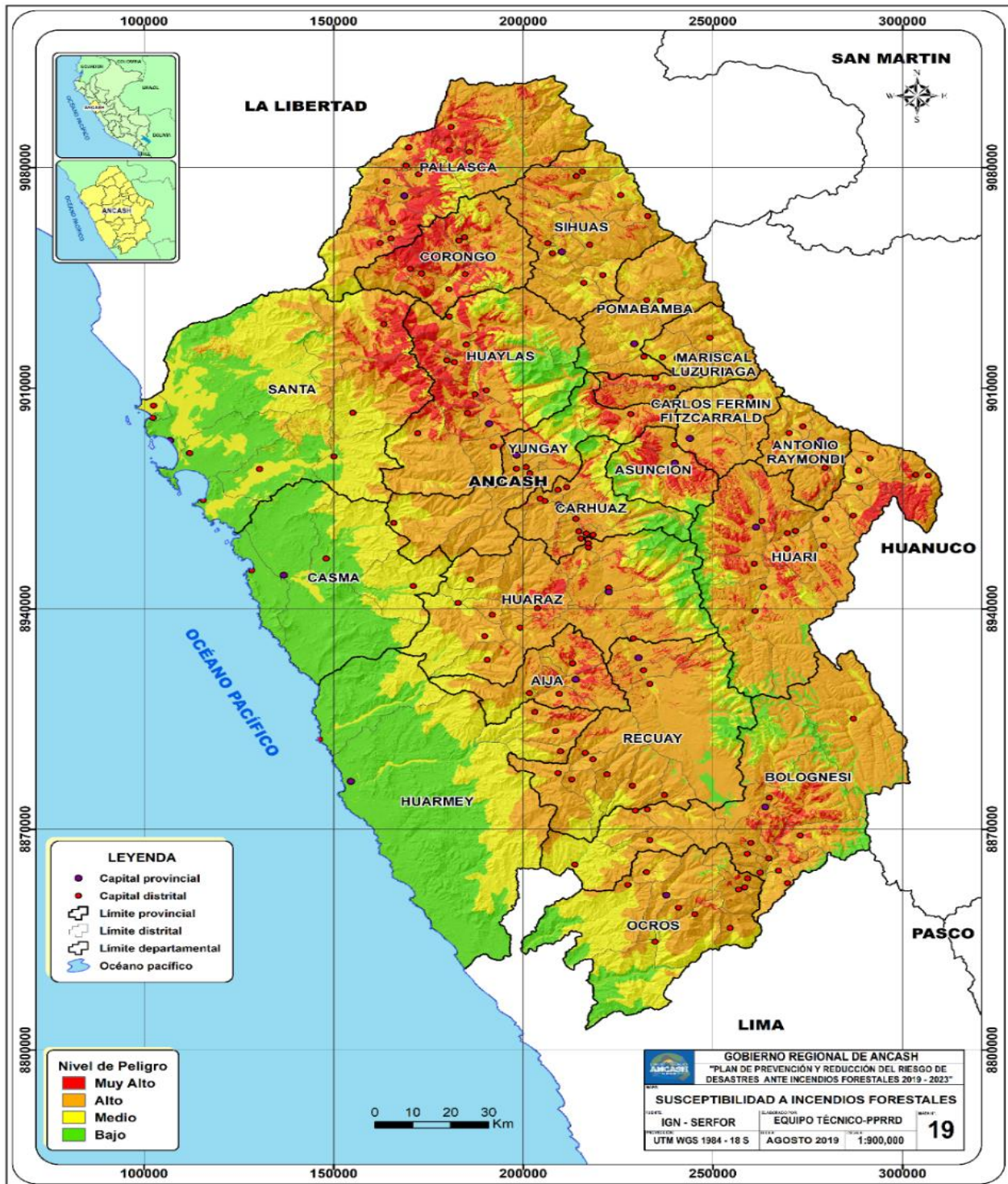
Mapa 41. Ancash: Susceptibilidad a incendios forestales
