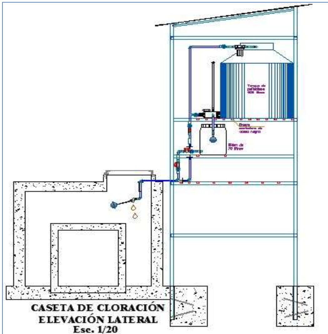
Imagen N° 02: Modelo M2 Equipo de Cloración Costado del Reservorio
